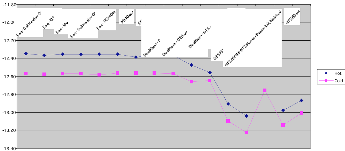
-12V EU [V]
